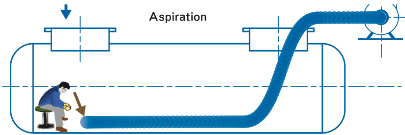
2a. Risque toxique - Ventilation par aspiration en présence d'un opérateur.
