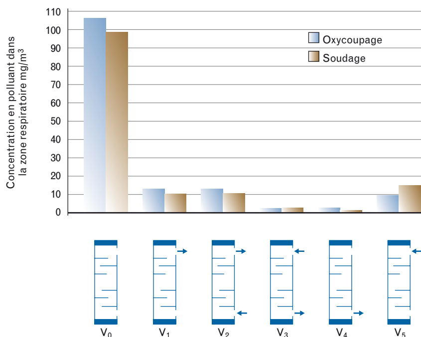
Fig. 3. Performances comparées de cinq schémas de ventilation pour soudage et oxycoupage au sol. Les flèches indiquent une aspiration ou un soufflage forcé (d'après : Guidelines for work in confined spaces - Exxon Corporation Medical Department).
